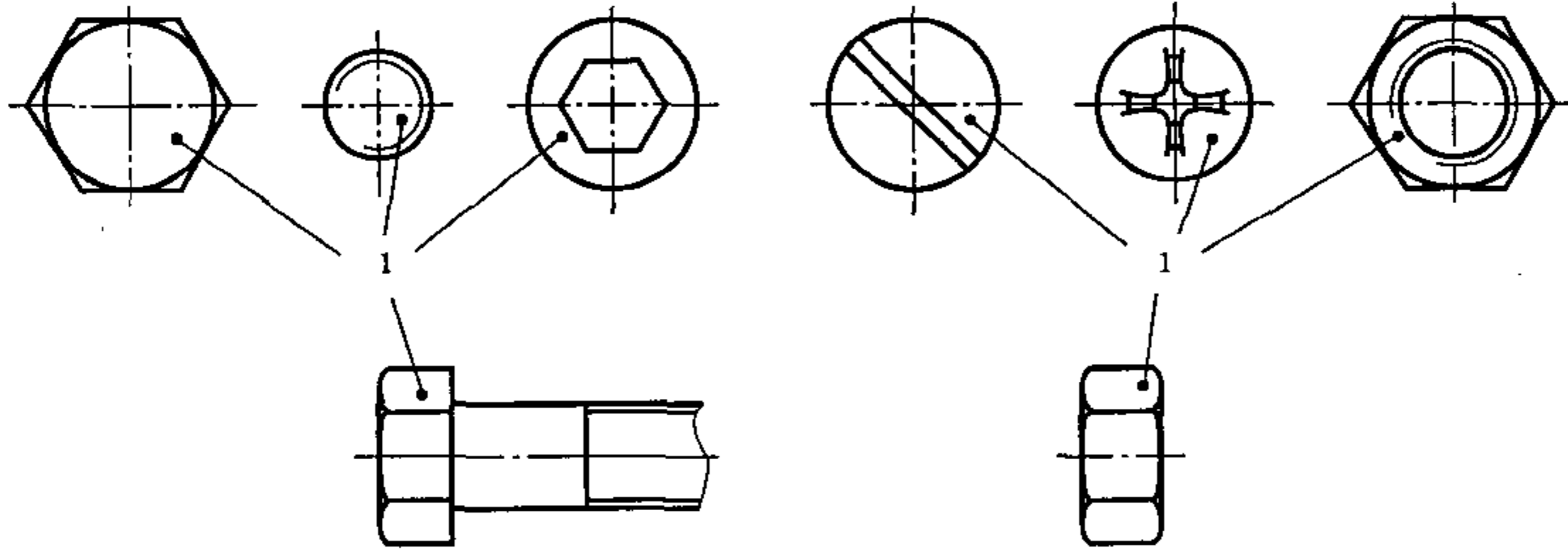
图 1 紧固件局部镀层厚度测量部位
